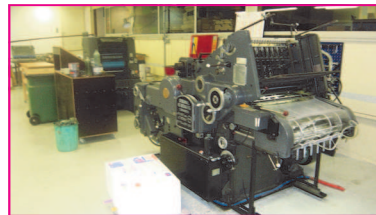
Ryobi quadrichromie 12000feuilles/heure format 36x52
