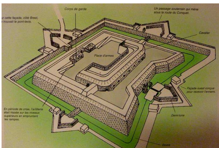
Maquette du fort à sa construction
